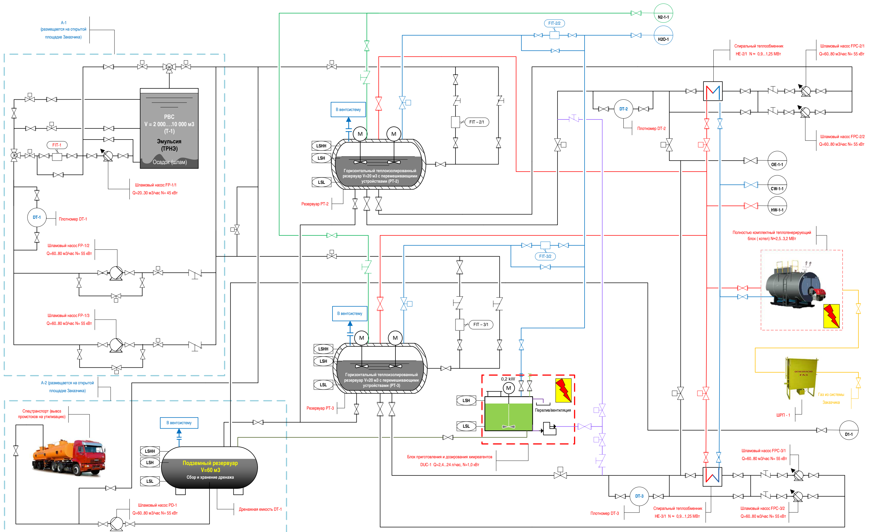
ЛИСТ 1. Участок подготовки эмульсии
